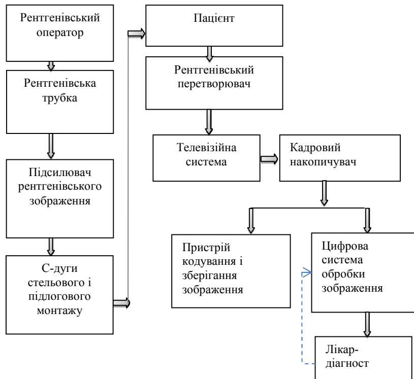
Рис. 1. Функціональна схема автоматизованої обробки ангиографічних зображень
